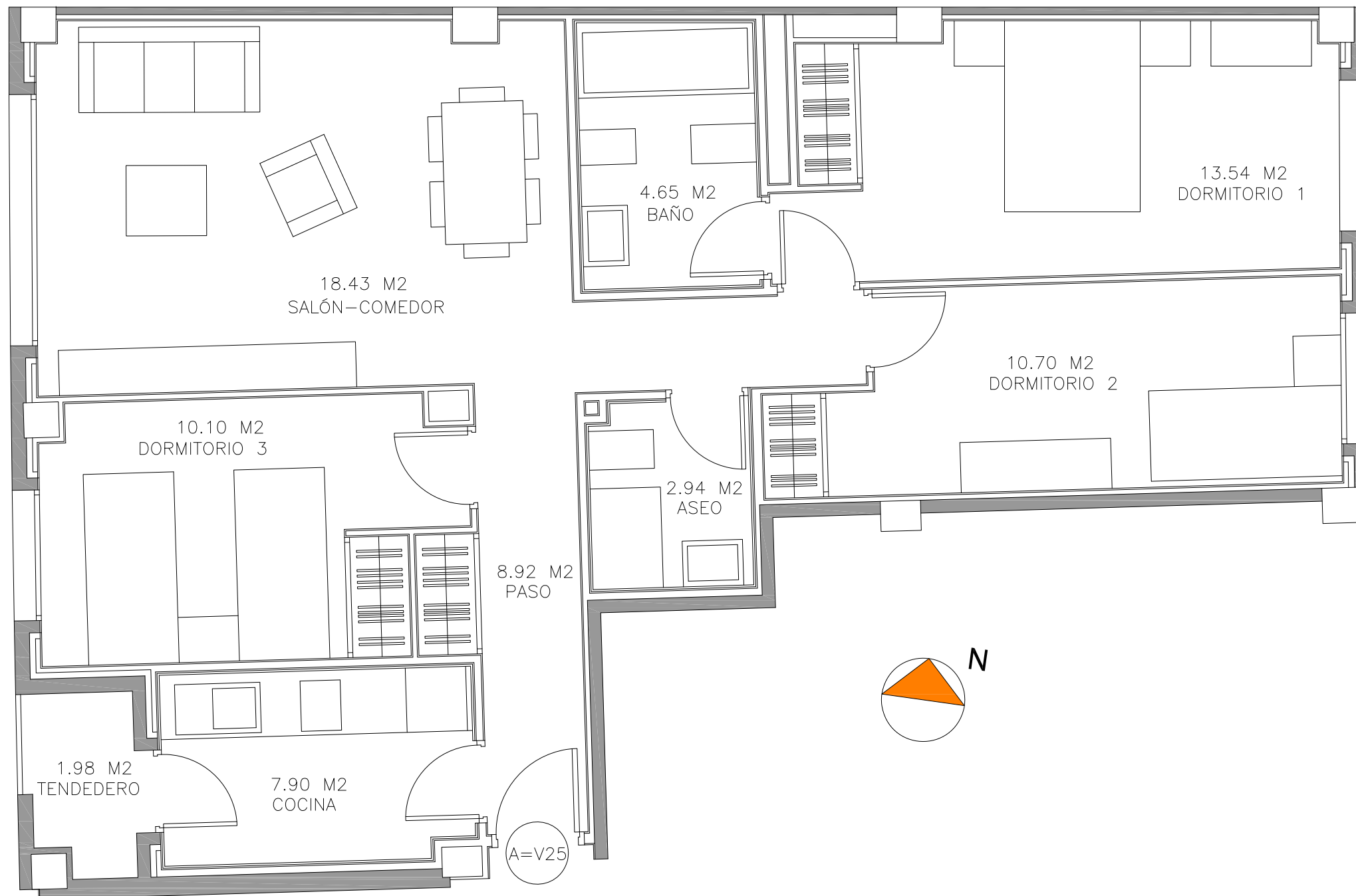
VIVIENDA TIPO V25
